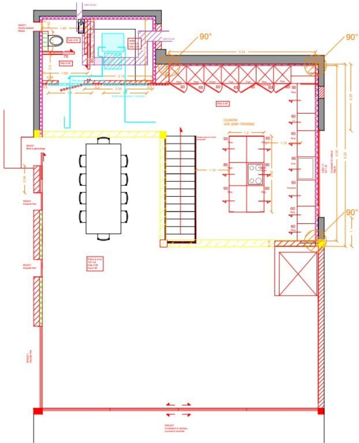
PLAN GÉNÉRAL R+2
